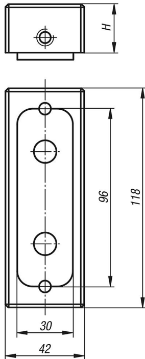
Elevação da altura do adaptador para o lado móvel
