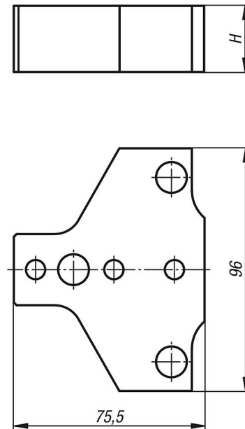
Elevação da altura do adaptador para o lado fixo
