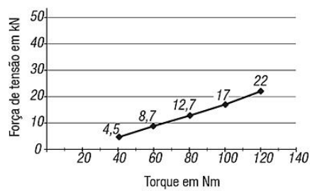
Força de tensão da morsa de 3 eixos
