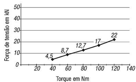
Força de tensão da morsa de 3 eixos
